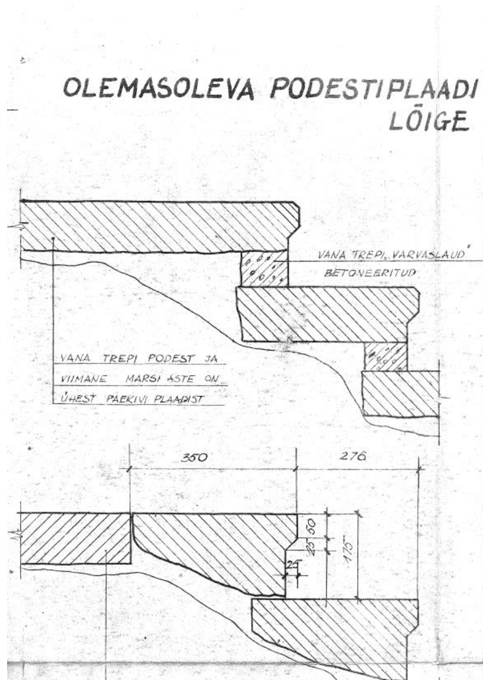
Joonis 4. Olemasoleva podestiplaadi lõige. (Eesti NSV MN Riikliku Ehituskomitee Vabariiklik Restaureerimisvalitsus, 1970)
