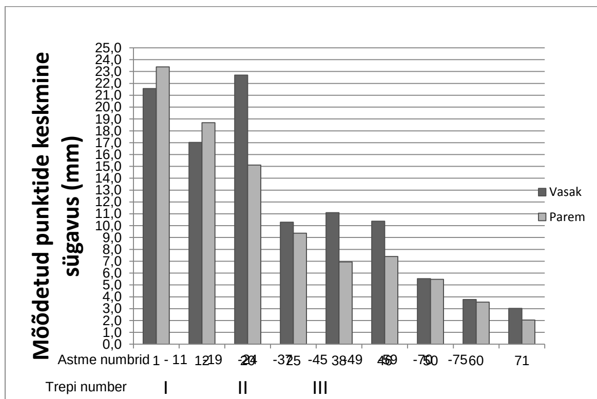
Joonis 12. GAGi peatrepi kulunud lohku keskmised väärtused trepikäikude kaupa
