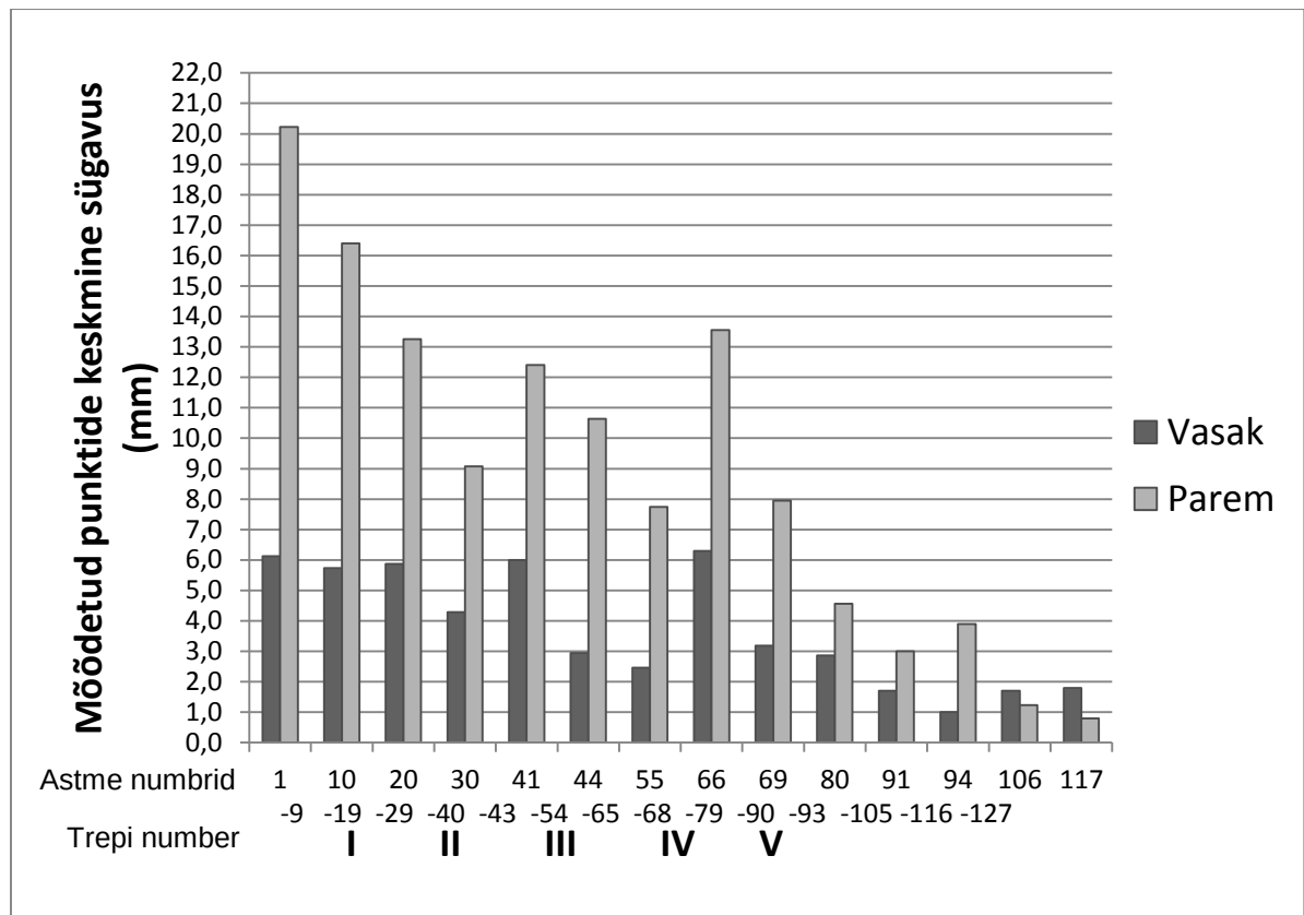
Joonis 13. Muinsuskaitseameti trepi kulunud lohku keskmine väärtused trepikäikude kaupa
